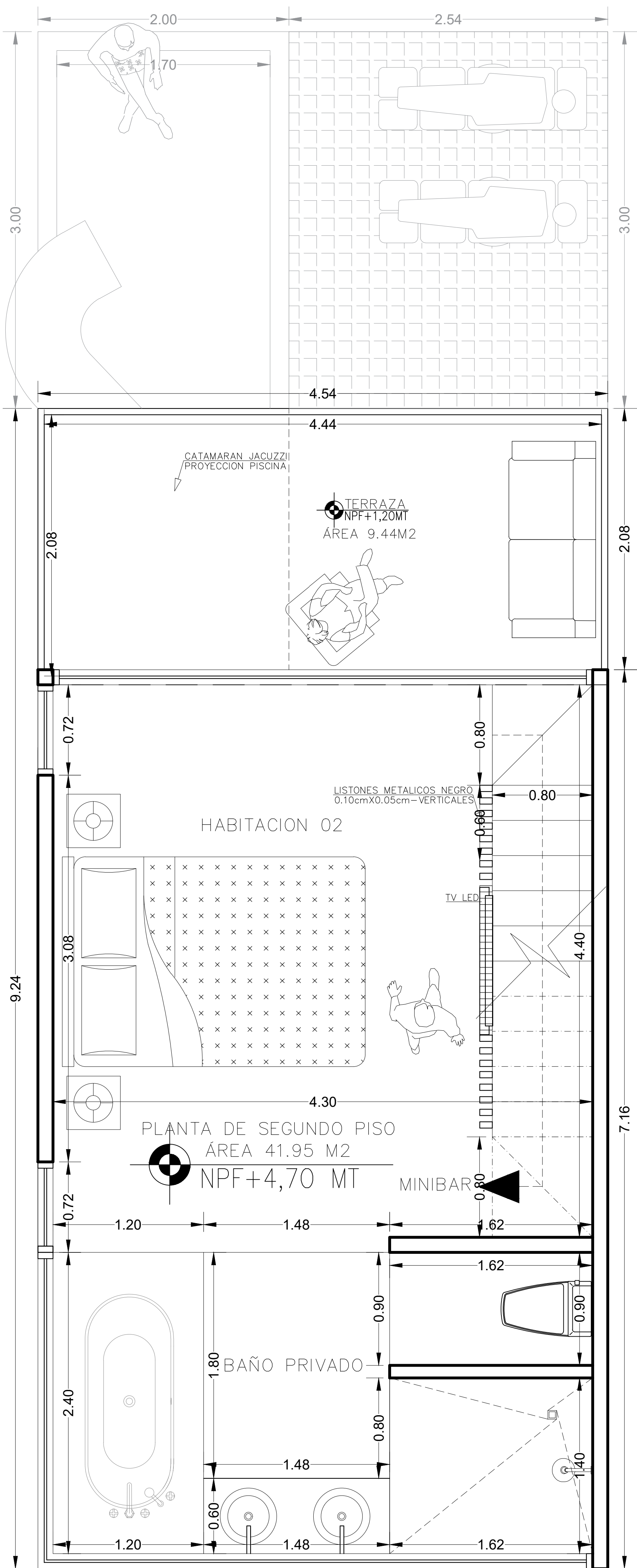
PLANTA 2 SUPER CABAÑA Escala 1/50
