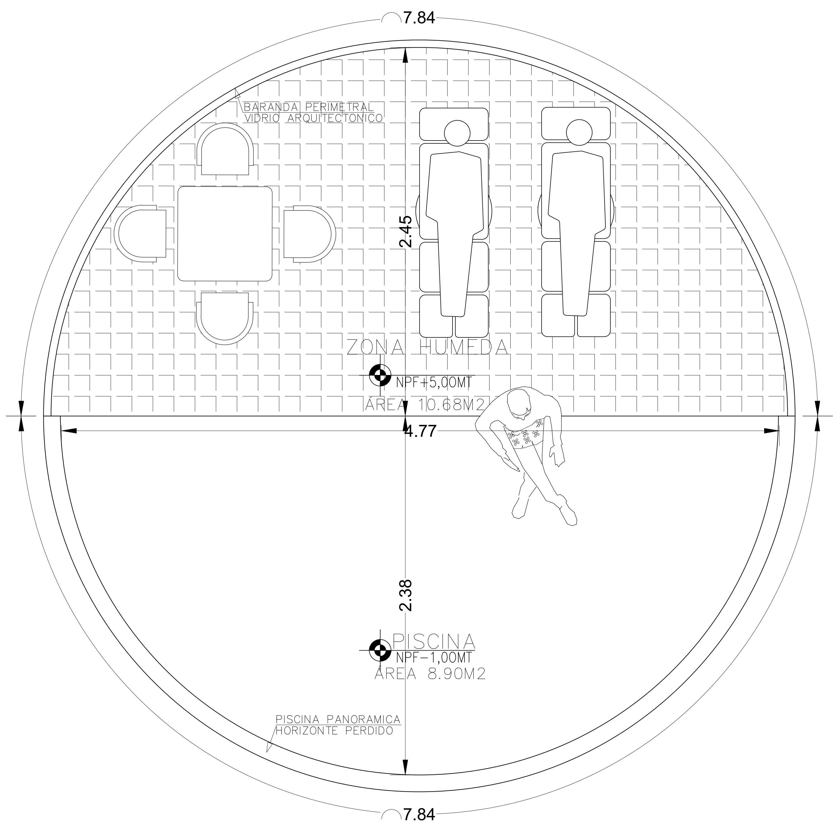
PLANTA SEGUNDO PISO CABAÑA Escala 1/50
