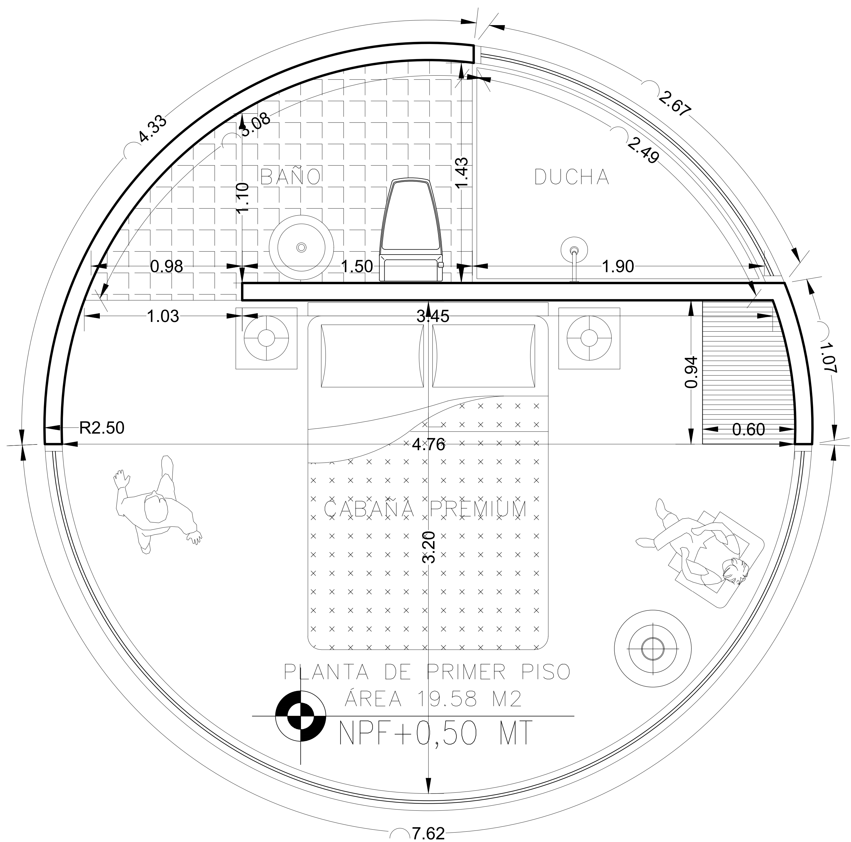
PLANTA PRIMER PISO CABAÑA Escala 1/50
