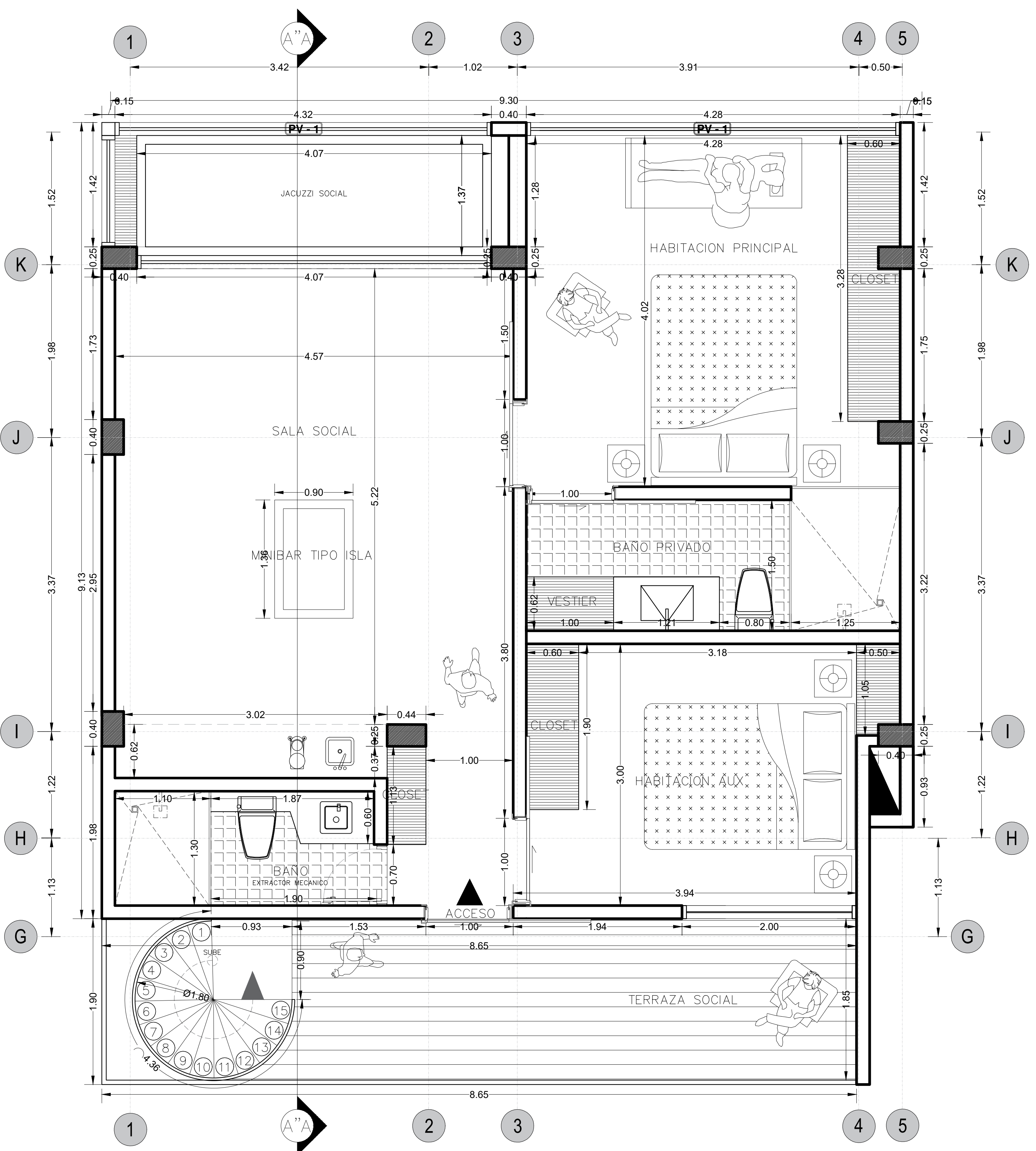
PLANTA MEZZANINE Escala 1/50
