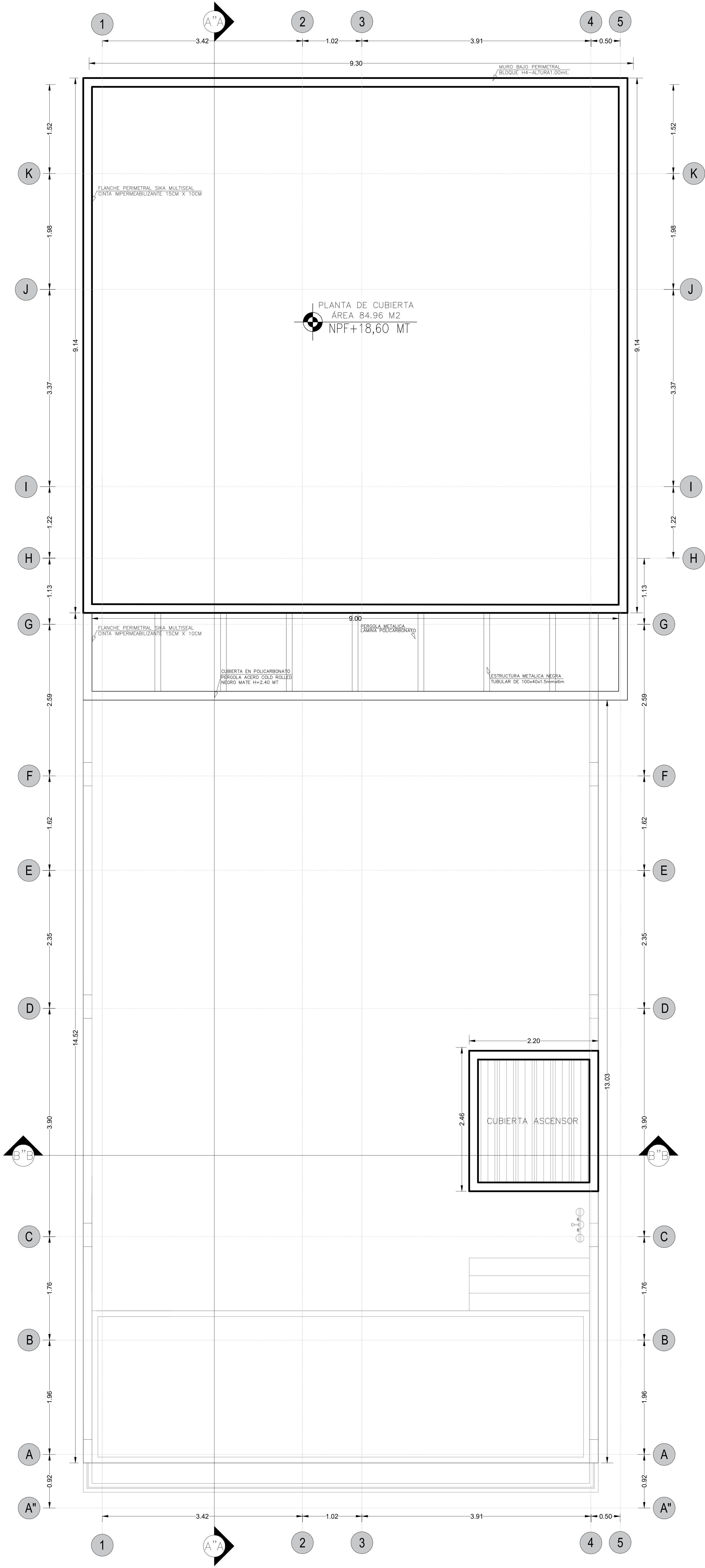
PLANTA DE CUBIERTA Escala 1/50
