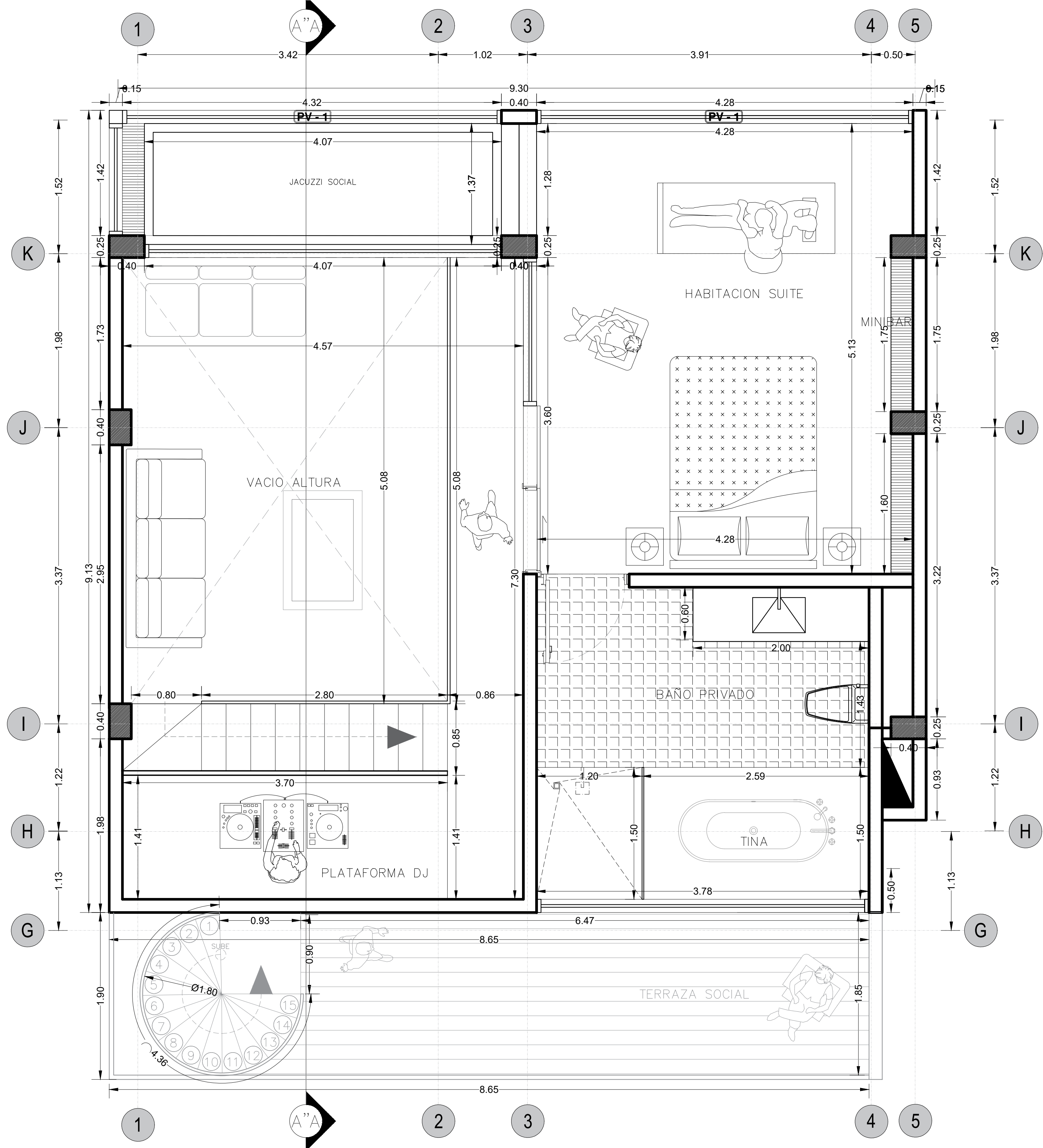
PLANTA MEZZANINE II Escala 1/50
